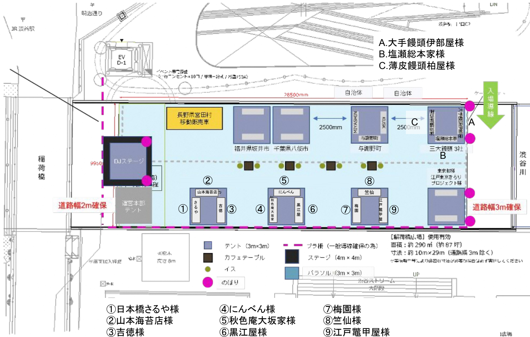
稲荷橋広場 基本図面 S = 1/100 (A3)
